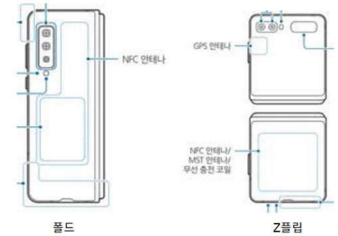
갤럭시 폴드 및 Z플립 NFC 위치
